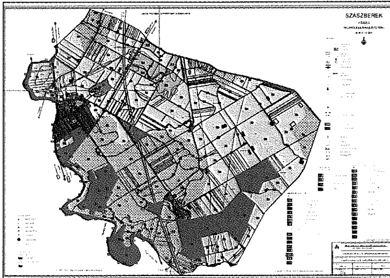
Településszerkezeti terv
